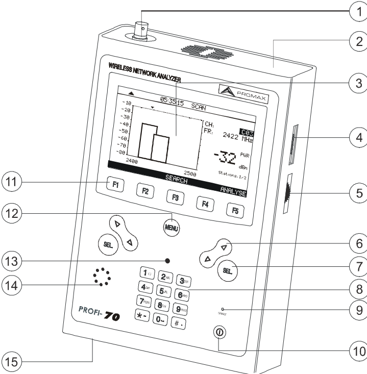
Figure 2.- Vue avant.
