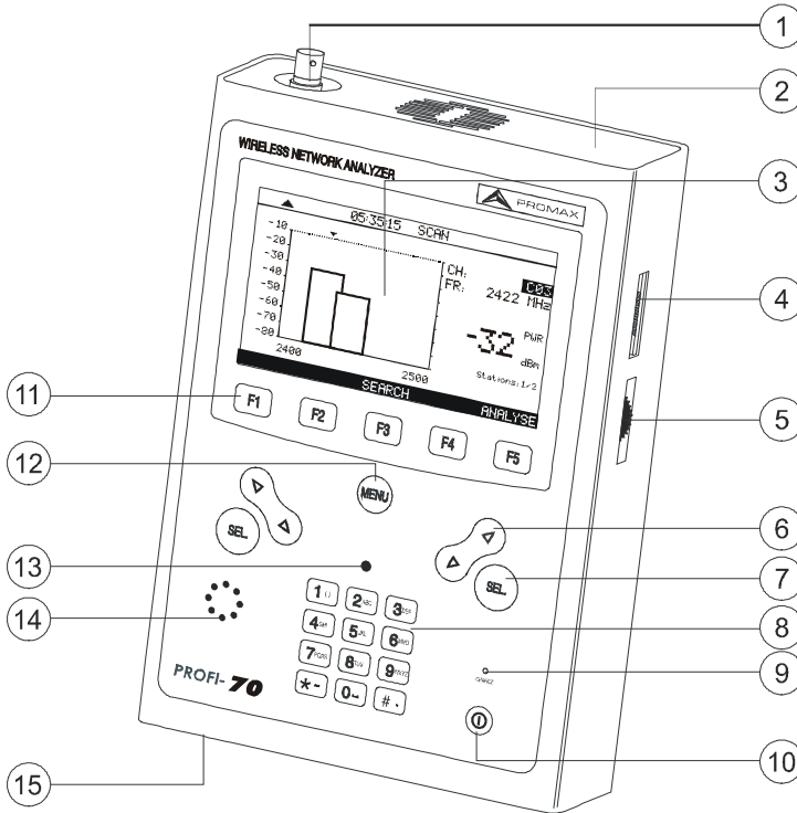
Figura 2.- Vista frontal
